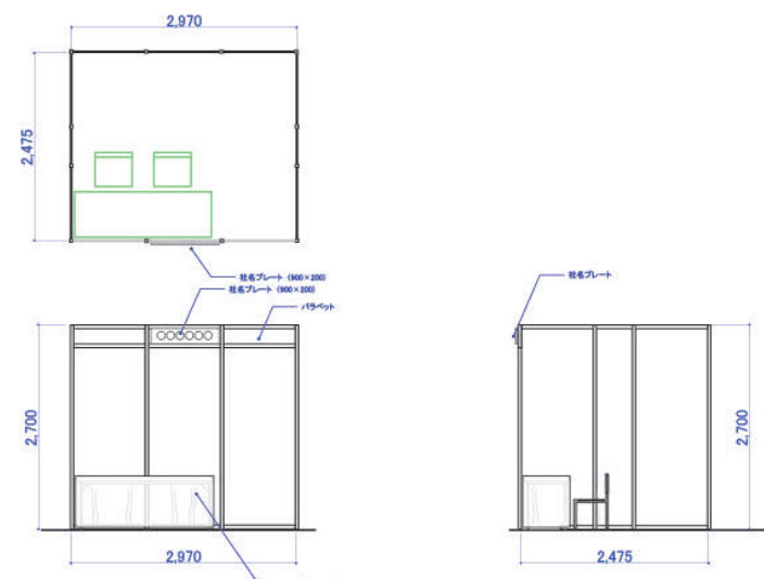
ブース詳細図 3m×2.5m
